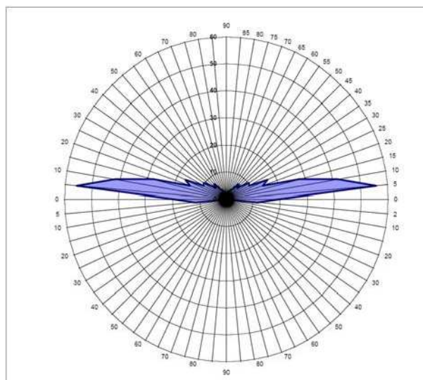
Obr.č.3 – Křivka svítivosti světelného zdroje LED s patičí E 27 v provedení RTO a OTL (bílý dioptř) dle ICAO (typ B, 32 cd)
