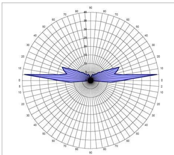
Obr.č.2 – Křivka svítivosti světelného zdroje LED s patičí E 27 v provedení RTO a OTL (červený dioptř) dle ICAO (typ A, 10 cd)
